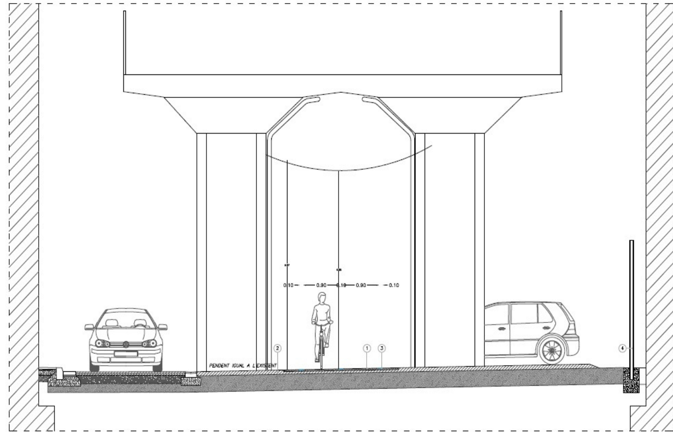
SECCIÓ CARRIL BICI EN APARCAMENT AMB ESPAI COMPARTIT AMB VEHICLES
